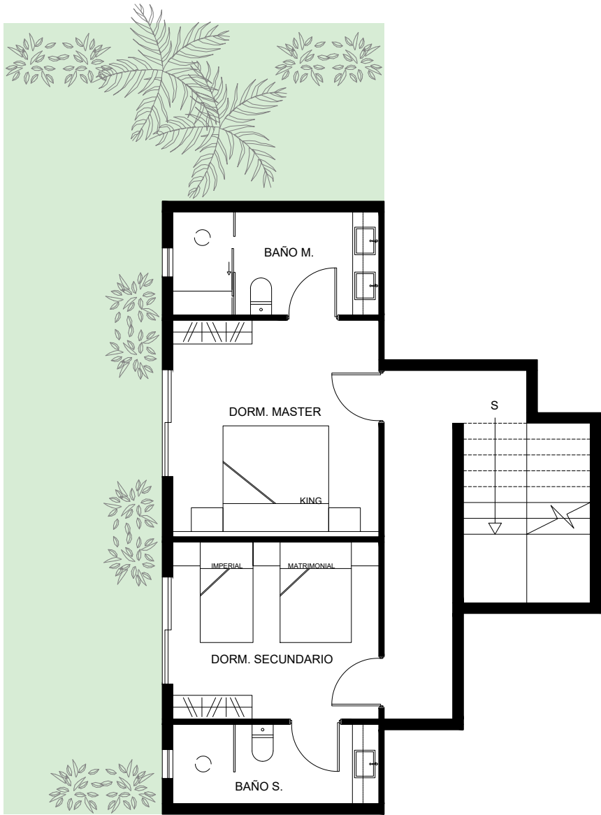
CASA B - PRIMER NIVEL
